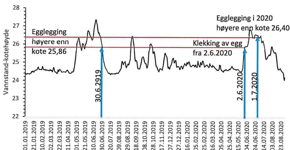
Fig. 3. Vannstand på Trøsken målestasjon i Kanal ovenfor Sølvstufoss i Ågårdselva for 1.1.2019 – 1.9.2020. Kote 25,86 er nedre grense for egg av tune flue funnet forsommer 2019, og egg som ligger fra kote 25,86 og videre oppover i elvebredden vanndekkes fra begynnelsen av juni 2020, betydelig senere enn i et normalår. Data fra Glommens og Laagens brukseierforening.
